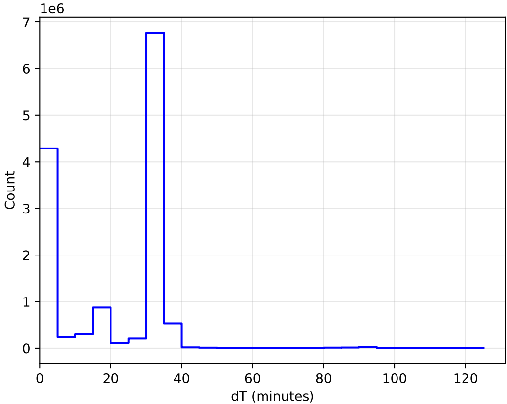
weather_cloudso35v3.4_10yrs All sky: DeltaT Histogram
