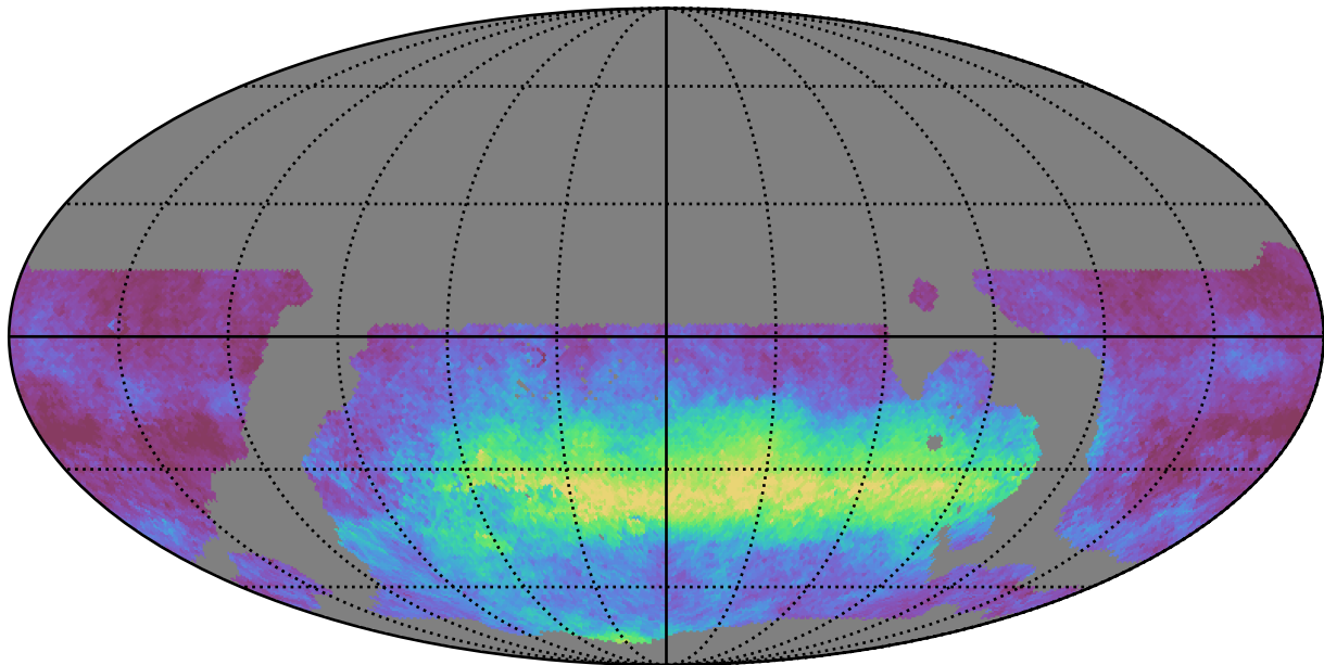
weather_cloudso35v3.4_10yrs WFD y band: AngleRms rotSkyPos
