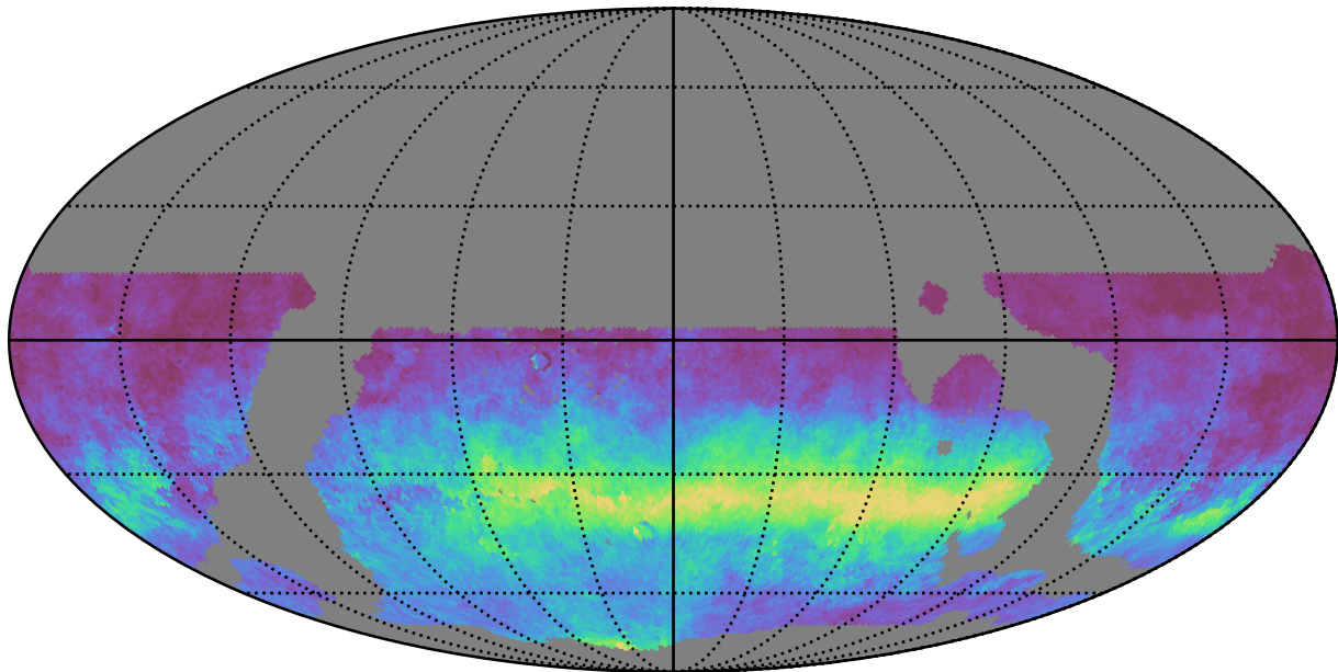
weather_cloudso35v3.4_10yrs WFD i band: AngleRms rotSkyPos
