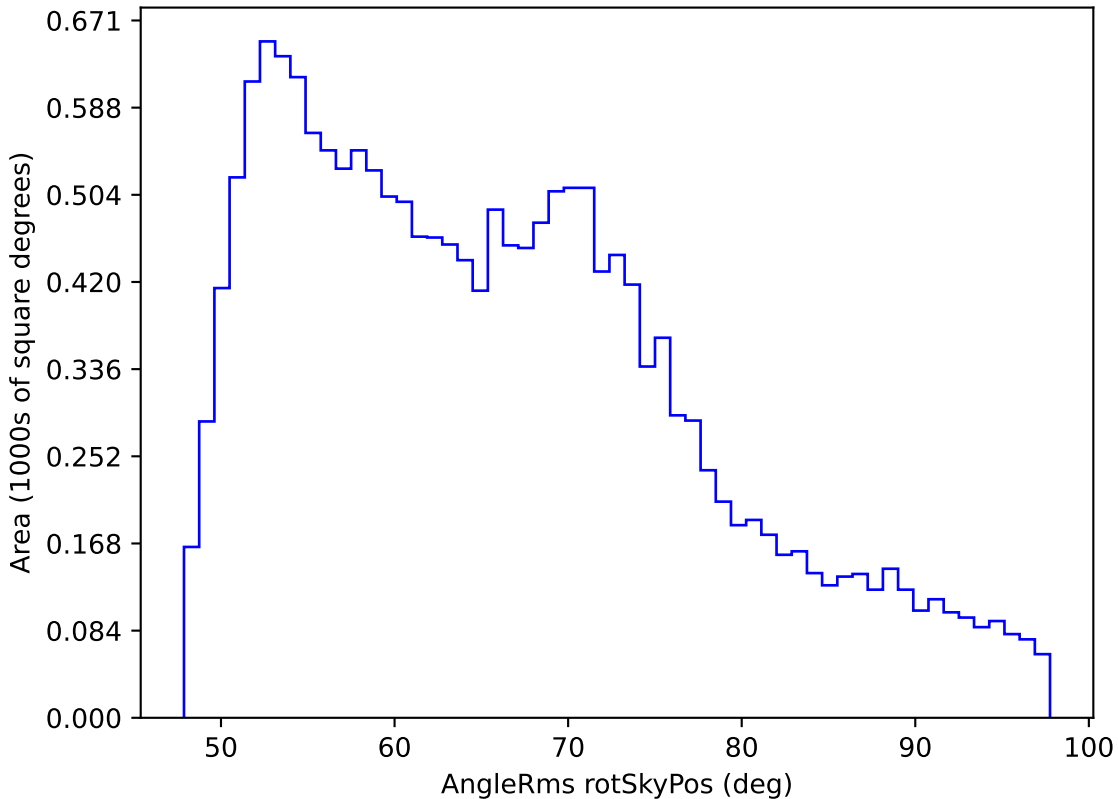
weather_cloudso35v3.4_10yrs WFD i band: AngleRms rotSkyPos
