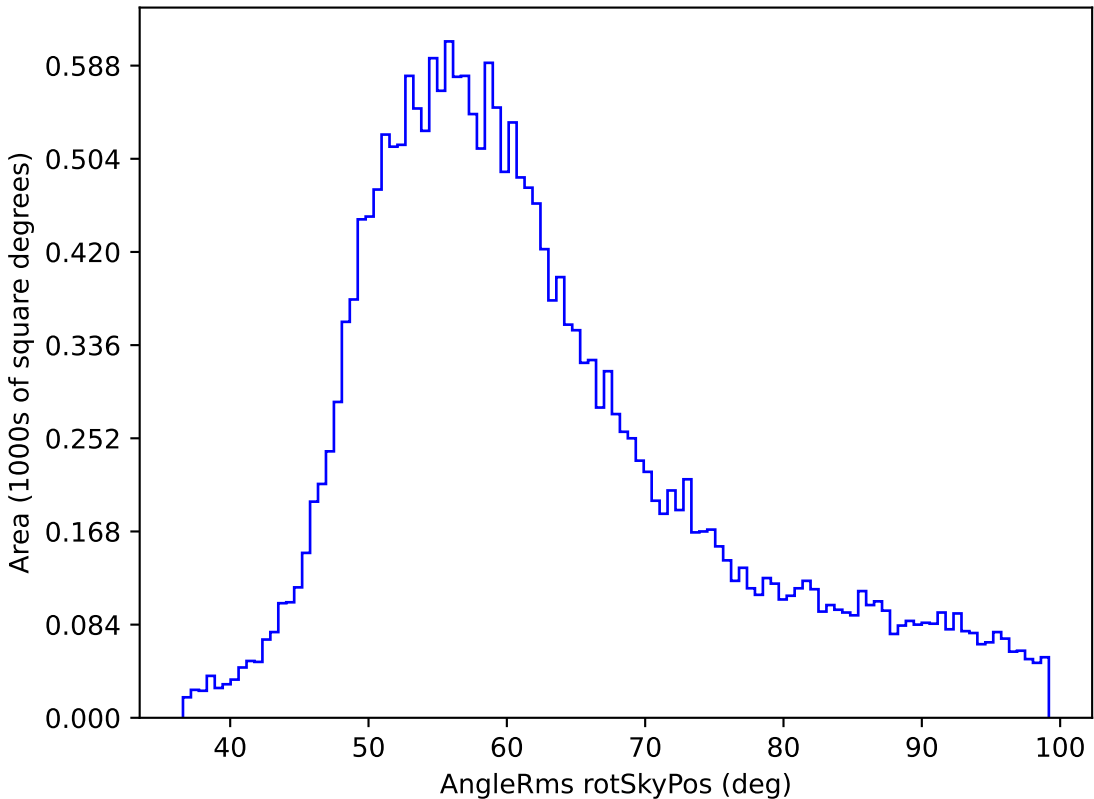
weather_cloudso35v3.4_10yrs All sky y band: AngleRms rotSkyPos
