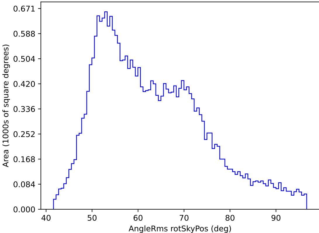
weather_cloudso35v3.4_10yrs All sky i band: AngleRms rotSkyPos
