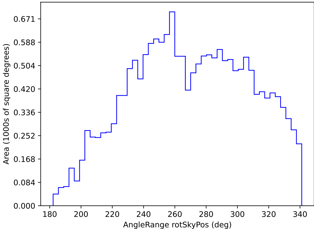
weather_cloudso35v3.4_10yrs WFD y band: AngleRange rotSkyPos
