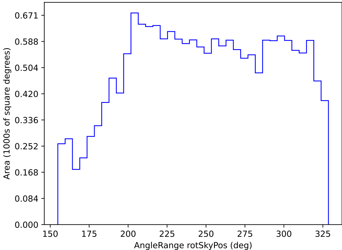
weather_cloudso35v3.4_10yrs WFD u band: AngleRange rotSkyPos
