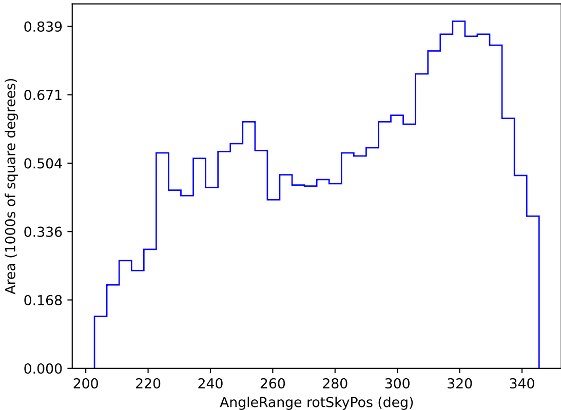
weather_cloudso35v3.4_10yrs WFD i band: AngleRange rotSkyPos
