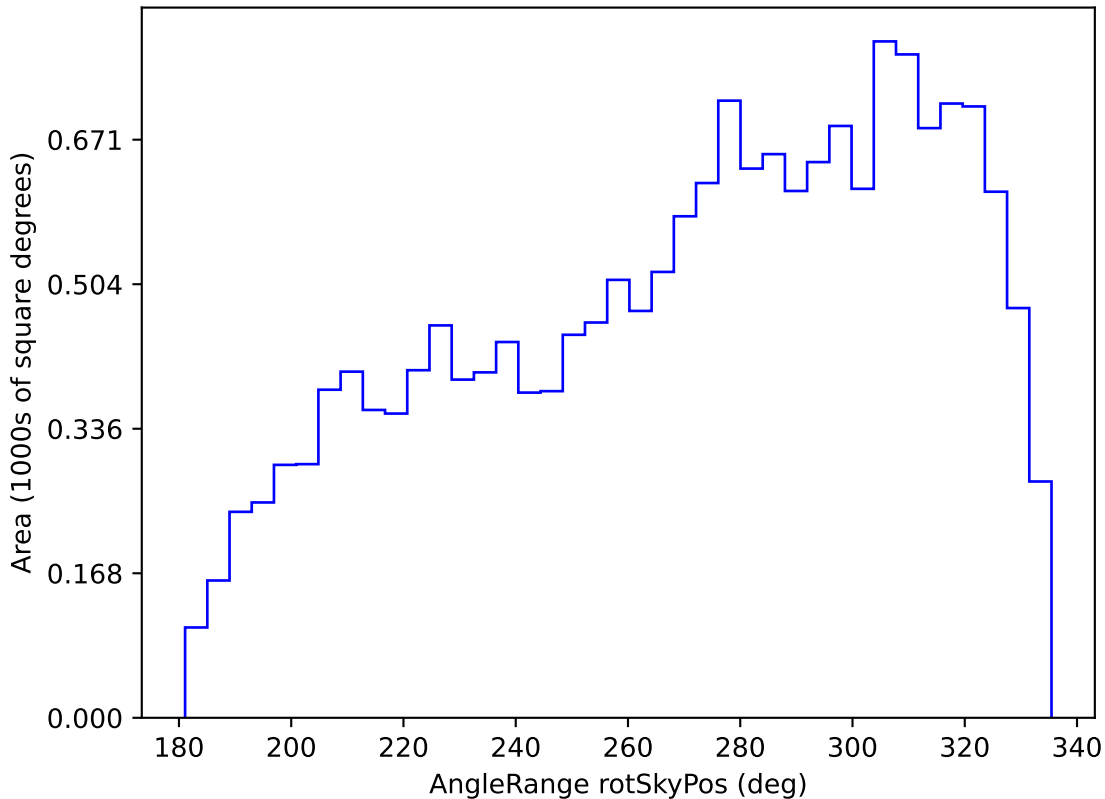
weather_cloudso35v3.4_10yrs WFD g band: AngleRange rotSkyPos
