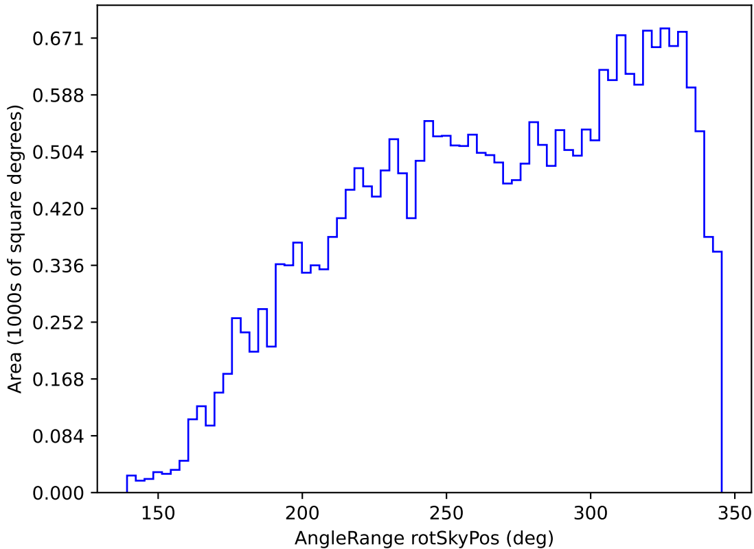
weather_cloudso35v3.4_10yrs All sky r band: AngleRange rotSkyPos
