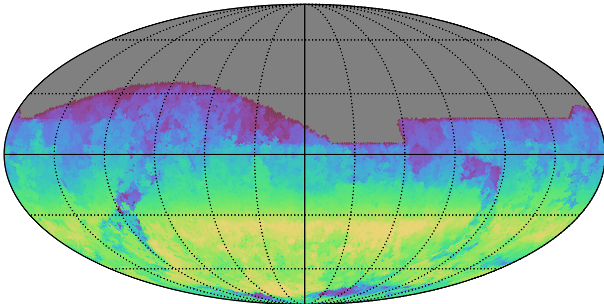
weather_cloudso35v3.4_10yrs All sky i band: AngleRange rotSkyPos
