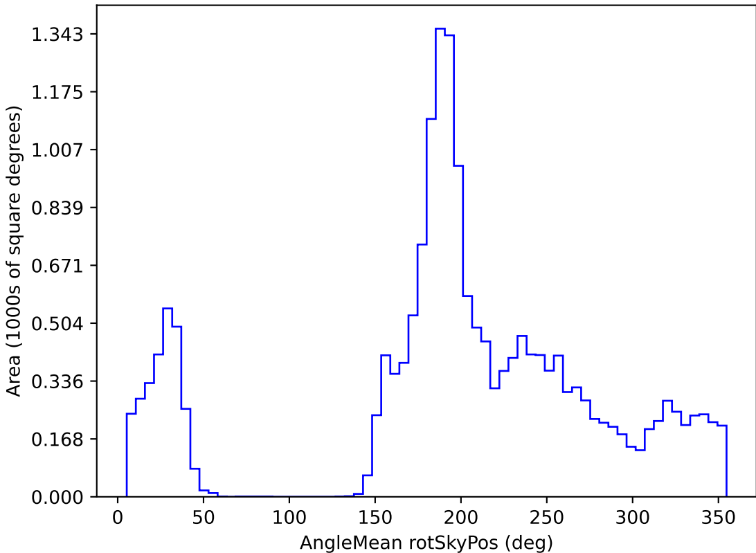
weather_cloudso35v3.4_10yrs WFD z band: AngleMean rotSkyPos
