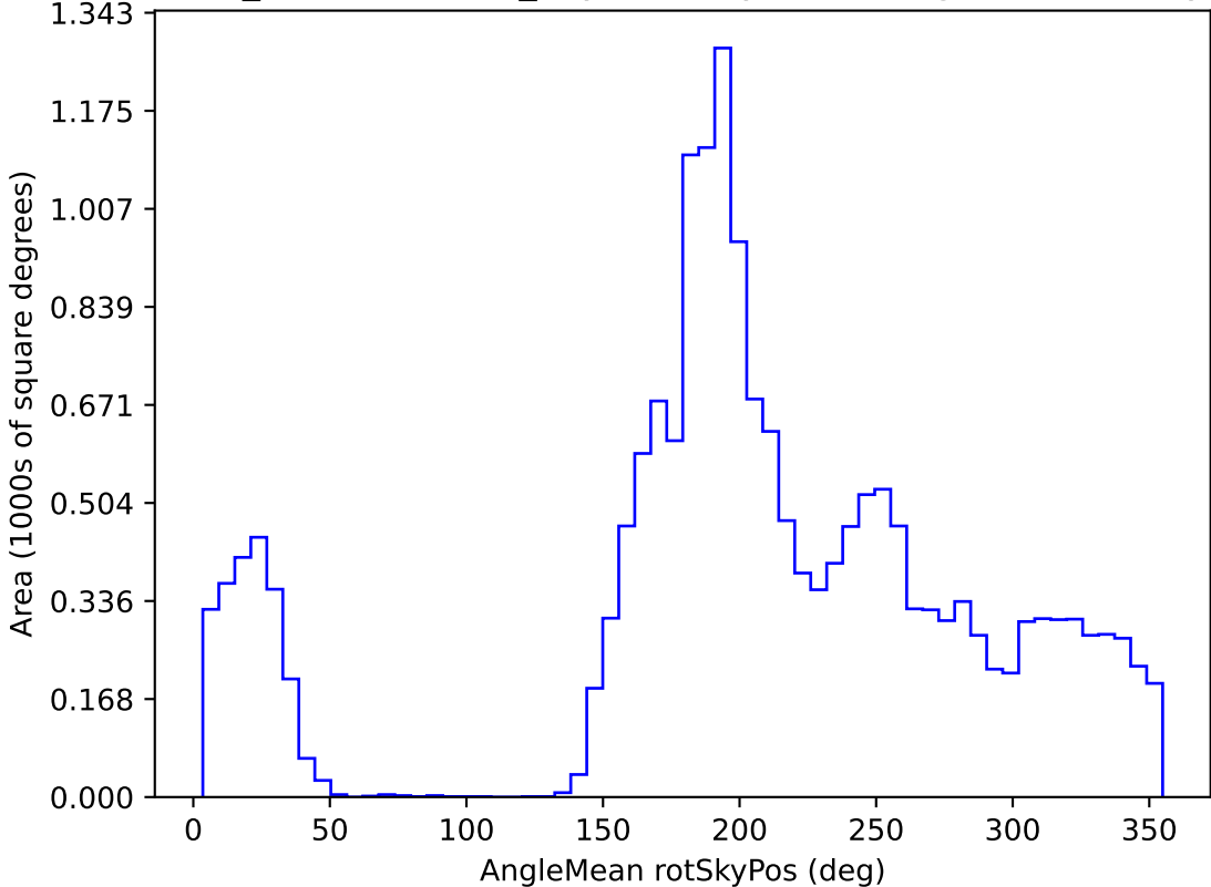
weather_cloudso35v3.4_10yrs WFD y band: AngleMean rotSkyPos
