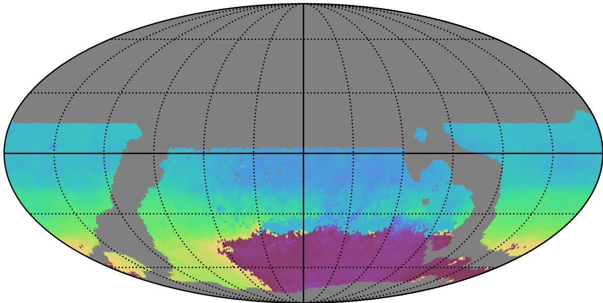
weather_cloudso35v3.4_10yrs WFD r band: AngleMean rotSkyPos
