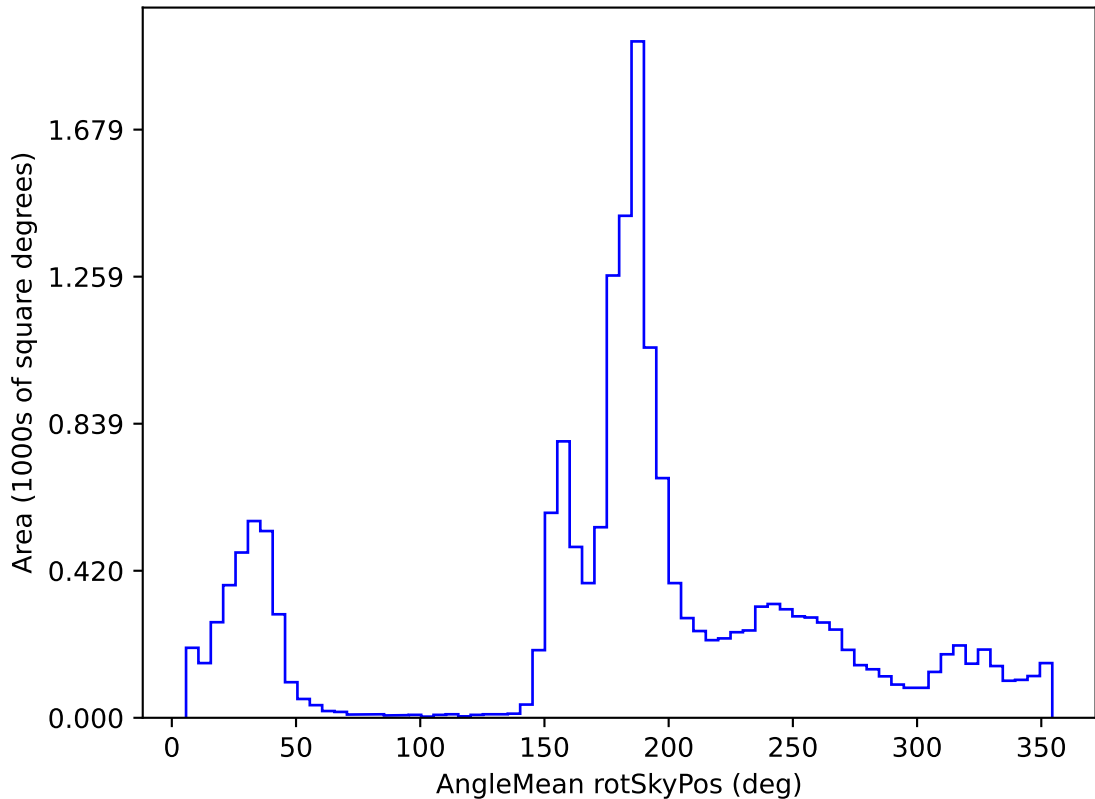
weather_cloudso35v3.4_10yrs WFD r band: AngleMean rotSkyPos
