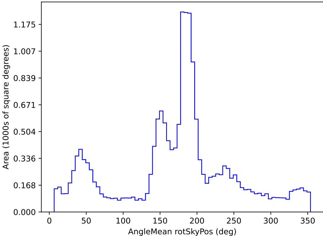
weather_cloudso35v3.4_10yrs WFD g band: AngleMean rotSkyPos
