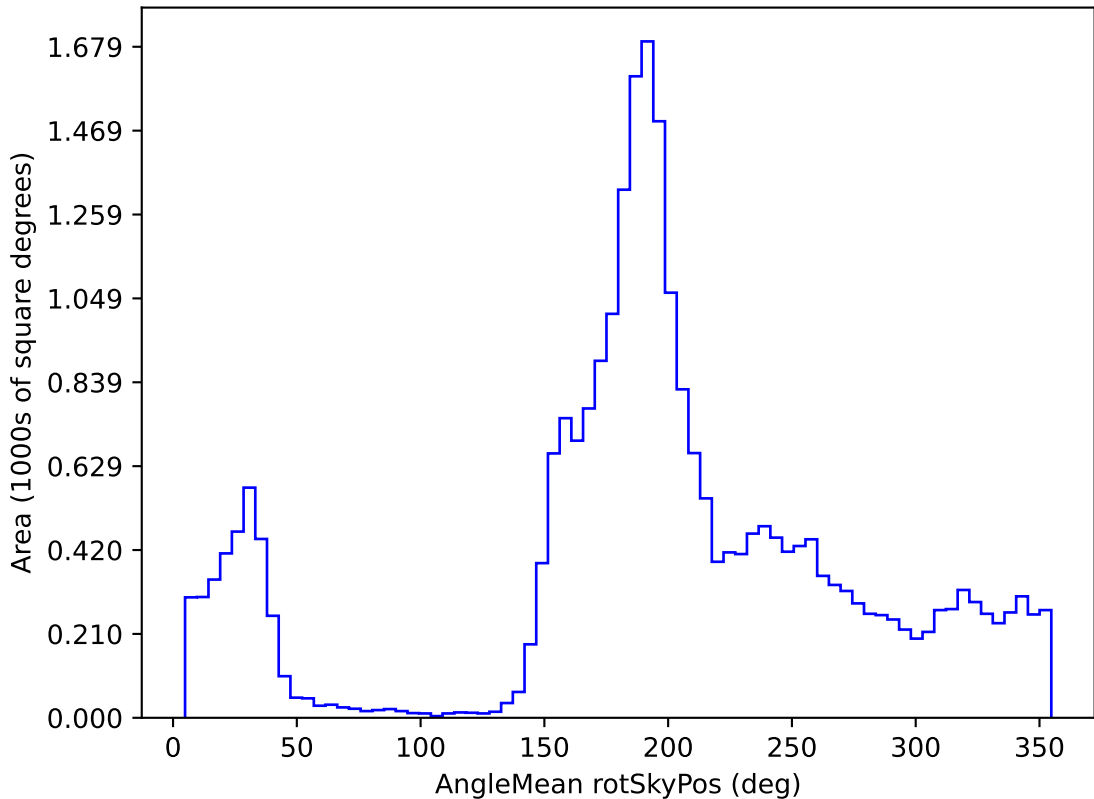
weather_cloudso35v3.4_10yrs All sky z band: AngleMean rotSkyPos
