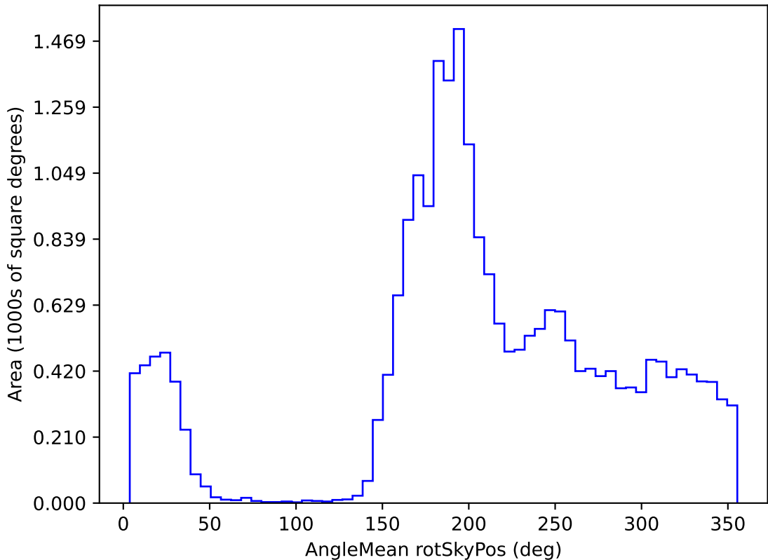
weather_cloudso35v3.4_10yrs All sky y band: AngleMean rotSkyPos
