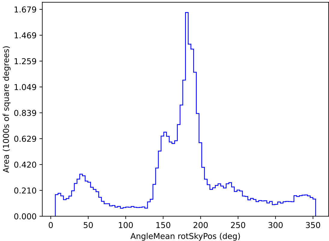
weather_cloudso35v3.4_10yrs All sky g band: AngleMean rotSkyPos
