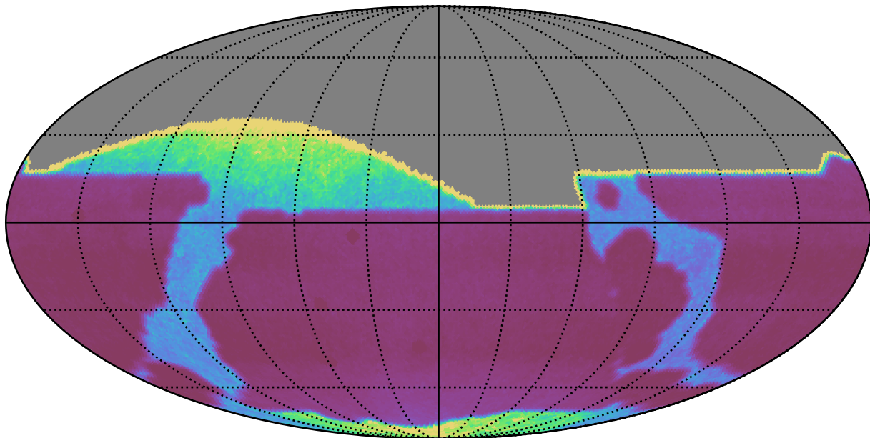
weather_cloudso35v3.4_10yrs : properMotion
