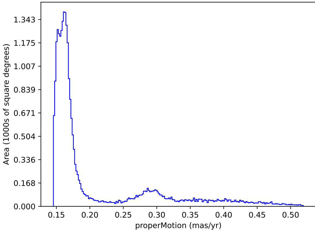
weather_cloudso35v3.4_10yrs : properMotion
