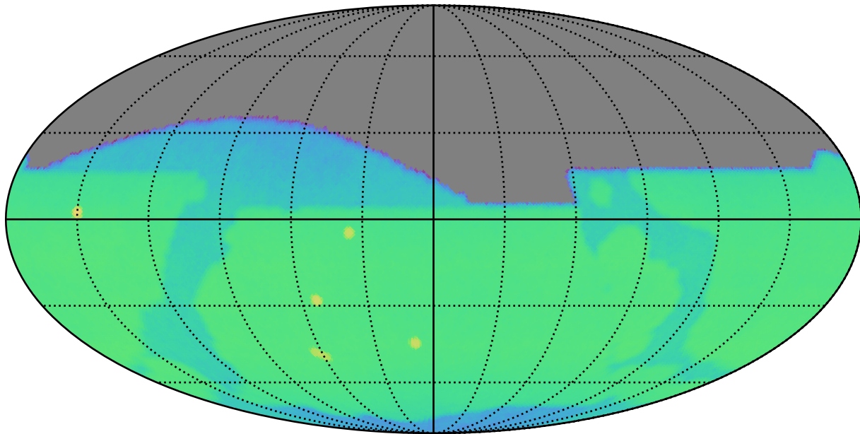
weather_cloudso35v3.4_10yrs i: CoaddM5
