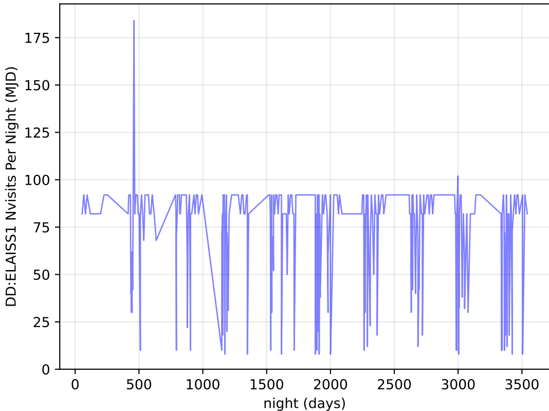
weather_cloudso35v3.4_10yrs all bands: DD:ELAISS1 Nvisits Per Night
