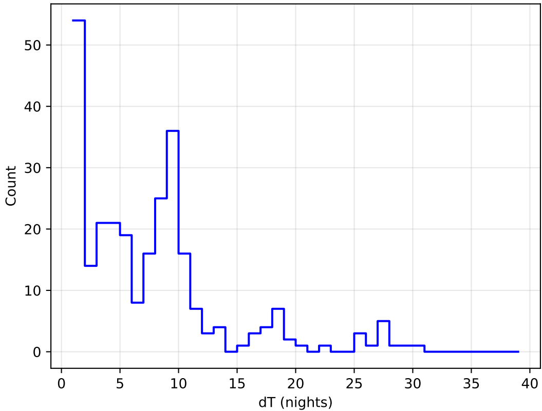
weather_cloudso35v3.4_10yrs all bands: DD:ELAISS1 Delta Nights Histogram
