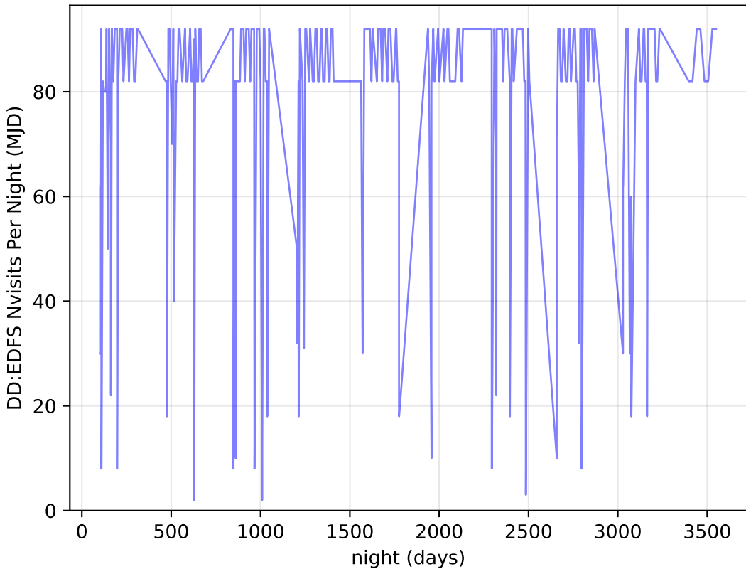
weather_cloudso35v3.4_10yrs all bands: DD:EDFS Nvisits Per Night
