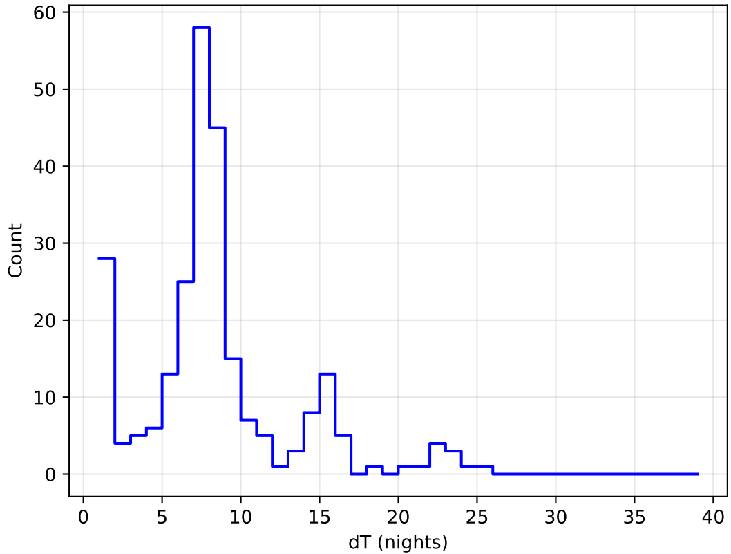
weather_cloudso35v3.4_10yrs all bands: DD:ECDFS Delta Nights Histogram
