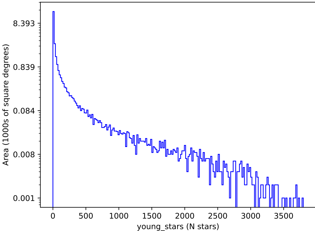
weather_cloudso31v3.4_10yrs : young_stars
