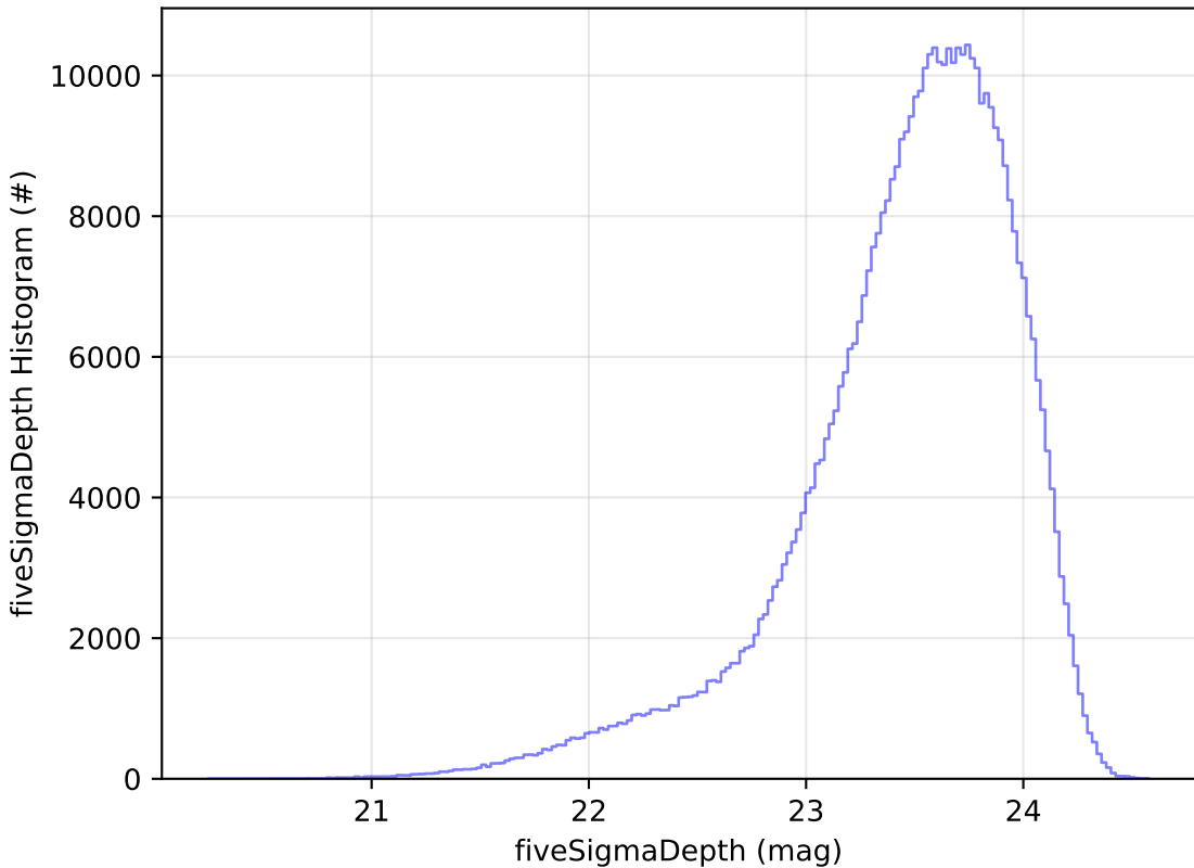
weather_cloudso31v3.4_10yrs i: fiveSigmaDepth Histogram
