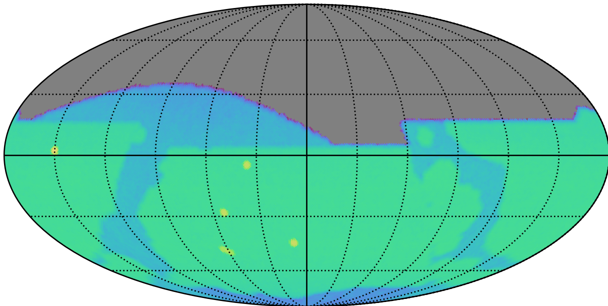
weather_cloudso31v3.4_10yrs i: SurfaceBrightLimit
