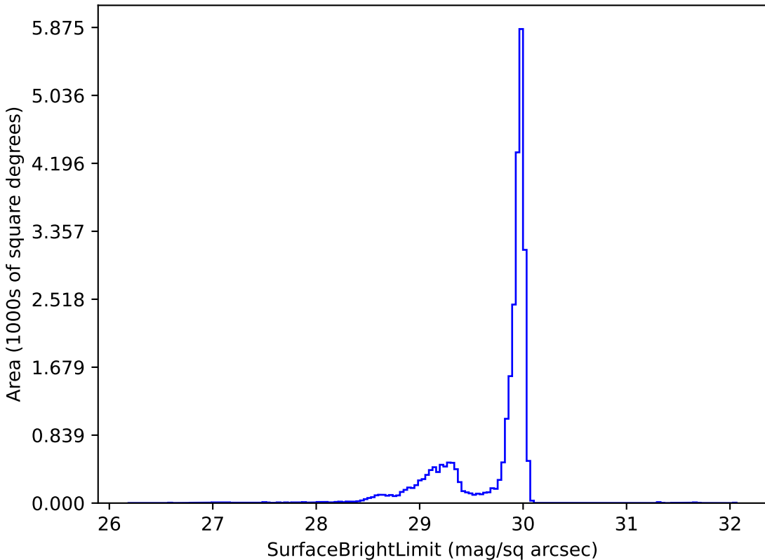
weather_cloudso31v3.4_10yrs i: SurfaceBrightLimit
