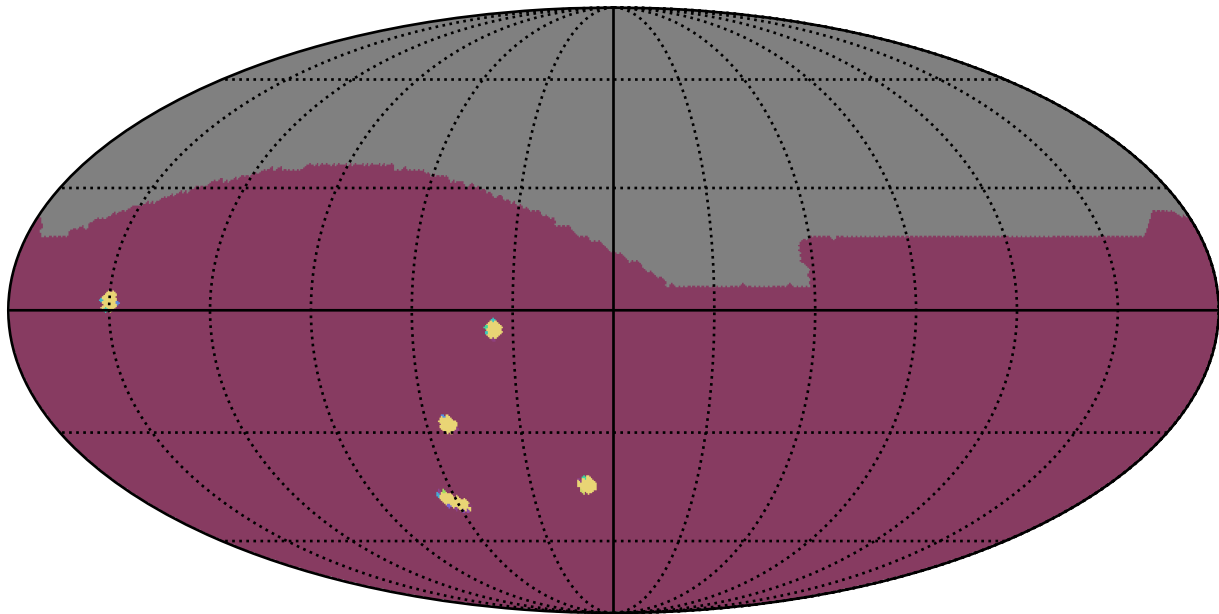
weather_cloudso31v3.4_10yrs : NumberOfQuickRevisits
