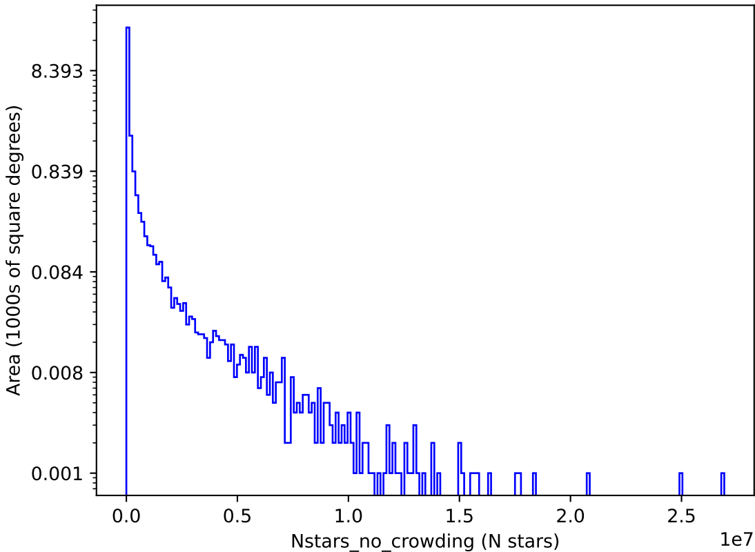
weather_cloudso31v3.4_10yrs z: Nstars_no_crowding
