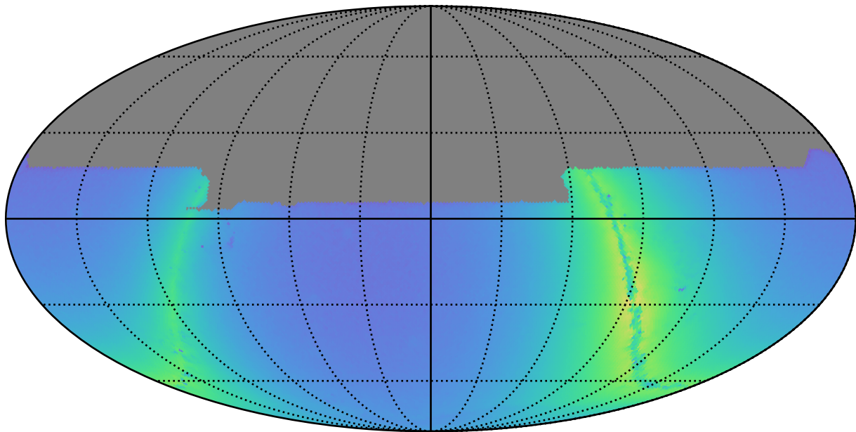
weather_cloudso31v3.4_10yrs y: Nstars_no_crowding
