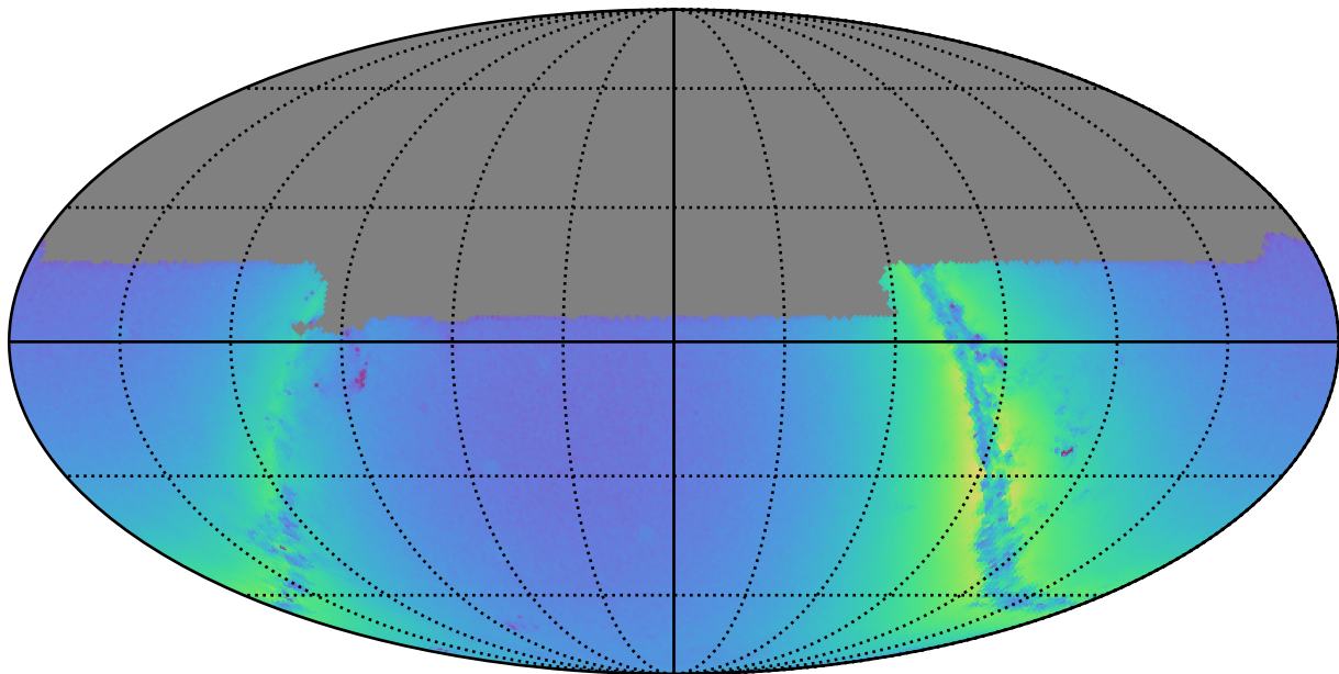
weather_cloudso31v3.4_10yrs u: Nstars_no_crowding
