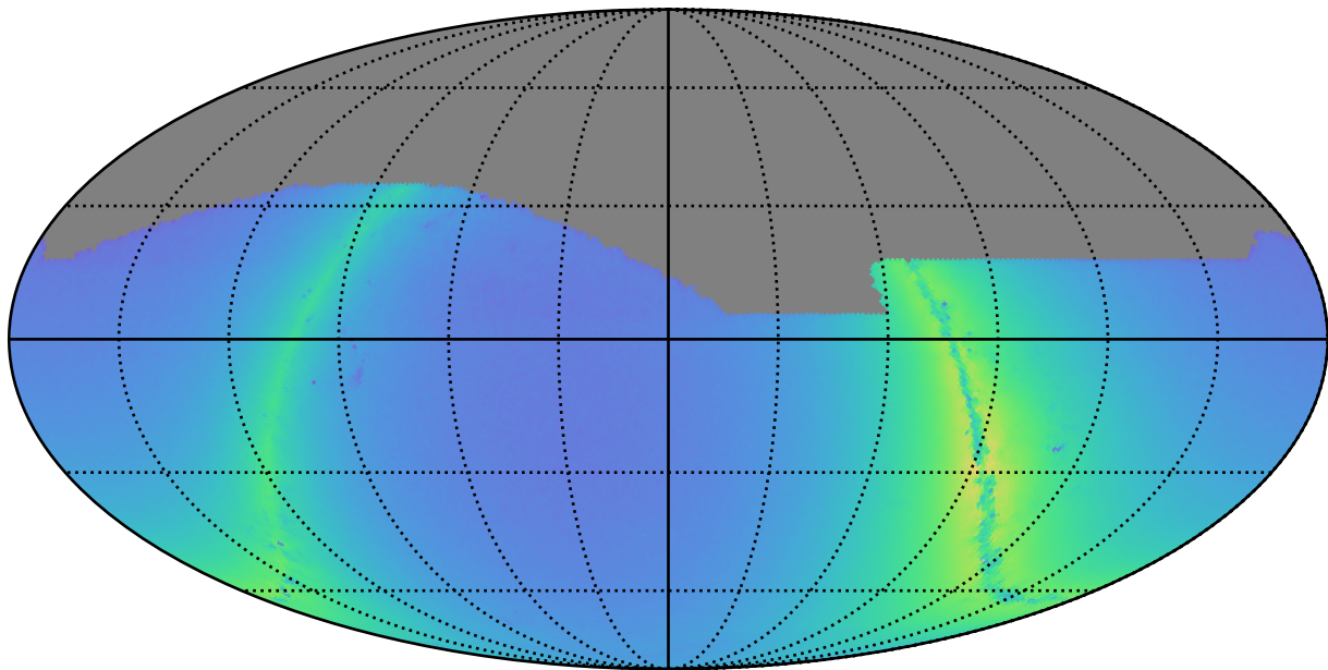
weather_cloudso31v3.4_10yrs i: Nstars_no_crowding
