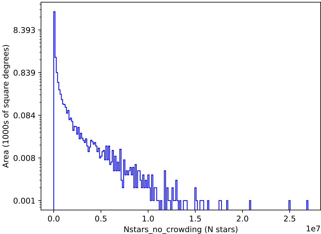
weather_cloudso31v3.4_10yrs i: Nstars_no_crowding
