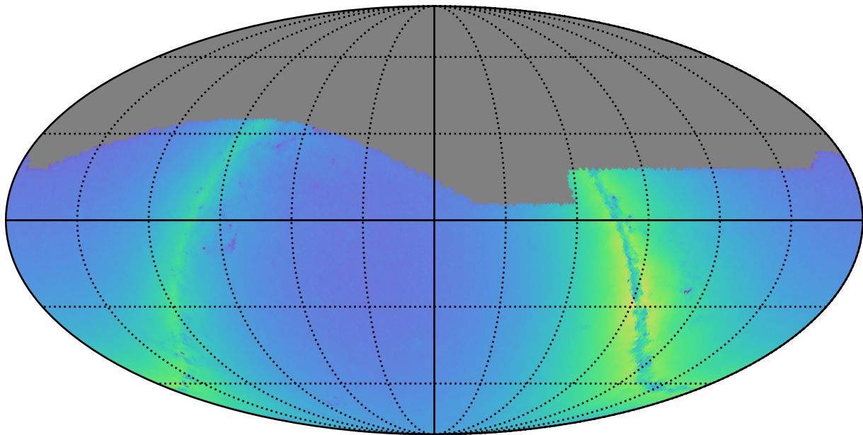
weather_cloudso31v3.4_10yrs g: Nstars_no_crowding
