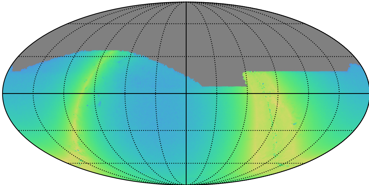
weather_cloudso31v3.4_10yrs i: N stars to Precision 0.20
