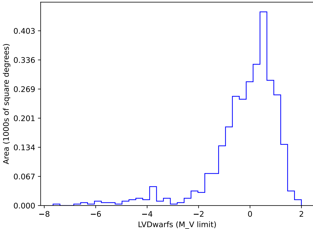
weather_cloudso31v3.4_10yrs gi SCP: LVDwarfs
