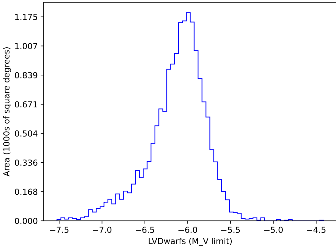
weather_cloudso31v3.4_10yrs gi: LVDwarfs
