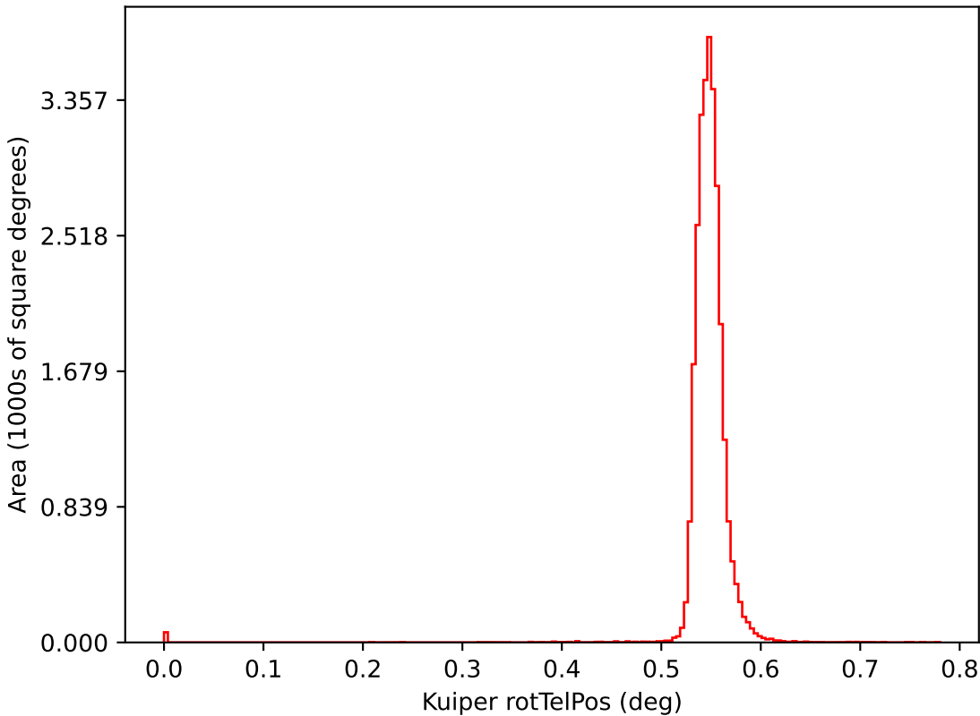
weather_cloudso31v3.4_10yrs i: Kuiper rotTelPos
