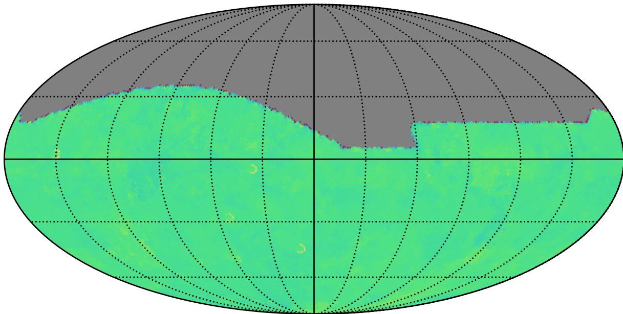
weather_cloudso31v3.4_10yrs g: Kuiper rotTelPos
