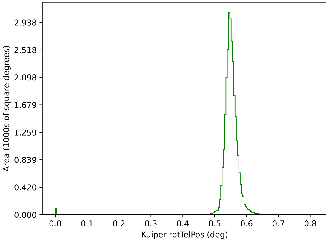
weather_cloudso31v3.4_10yrs g: Kuiper rotTelPos
