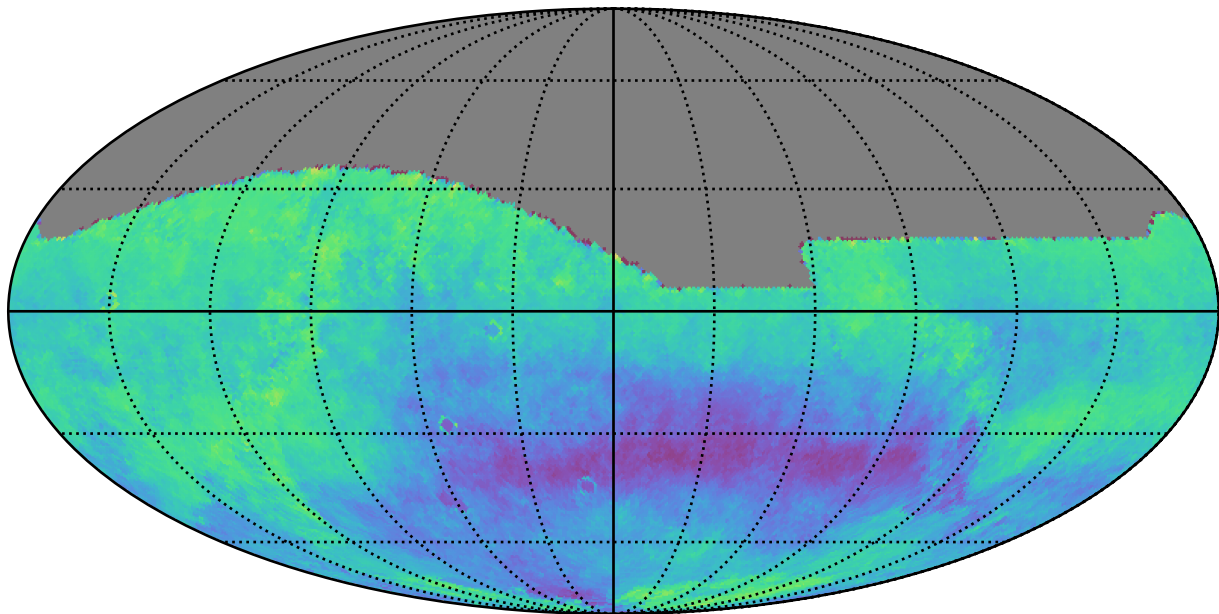
weather_cloudso31v3.4_10yrs z: Kuiper rotSkyPos
