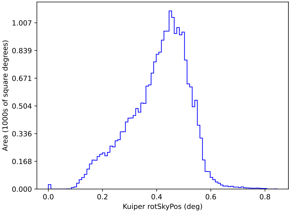
weather_cloudso31v3.4_10yrs y: Kuiper rotSkyPos
