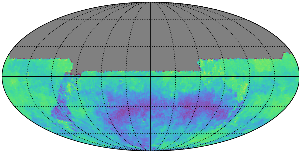
weather_cloudso31v3.4_10yrs u: Kuiper rotSkyPos
