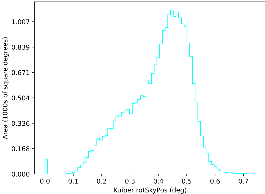
weather_cloudso31v3.4_10yrs u: Kuiper rotSkyPos
