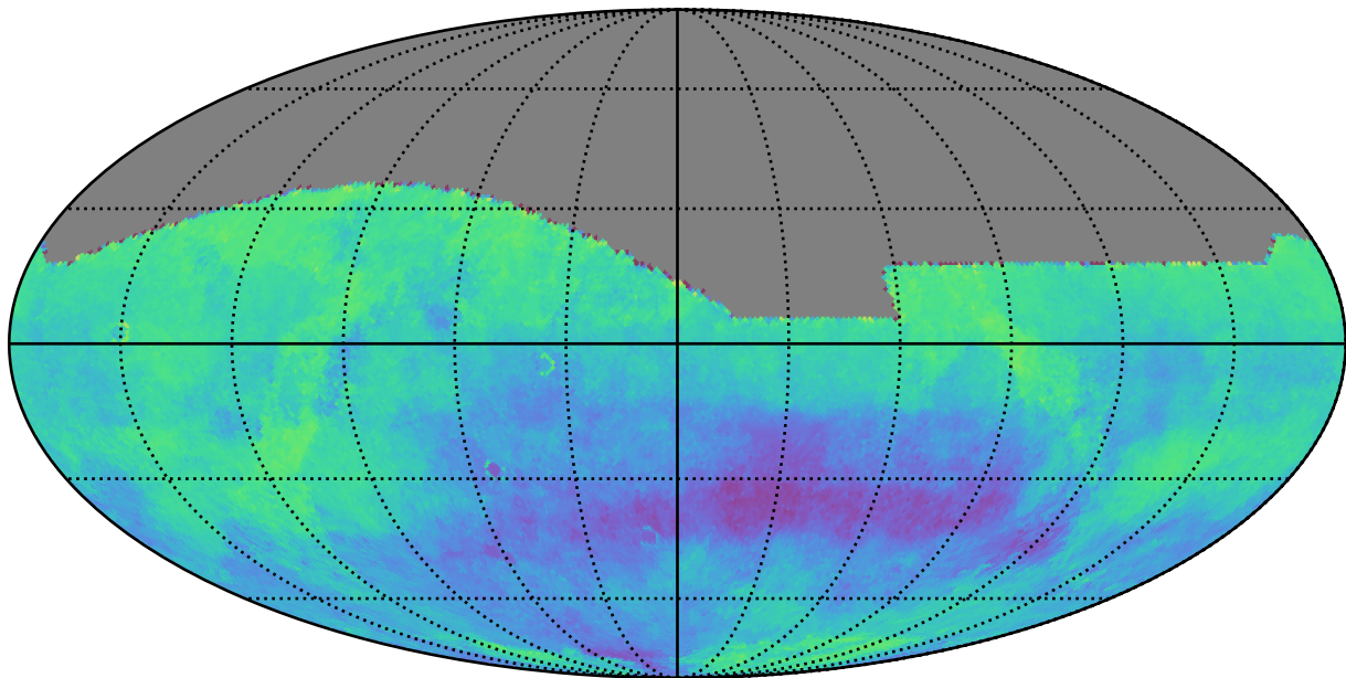
weather_cloudso31v3.4_10yrs i: Kuiper rotSkyPos
