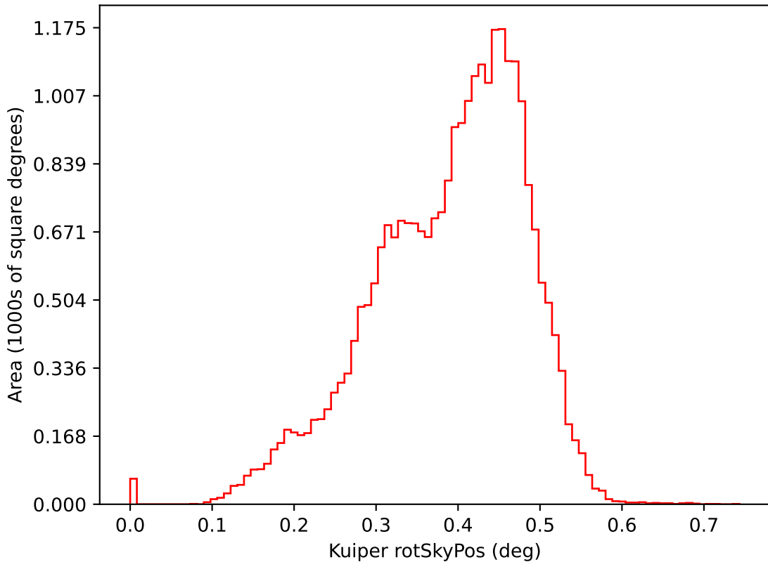
weather_cloudso31v3.4_10yrs i: Kuiper rotSkyPos
